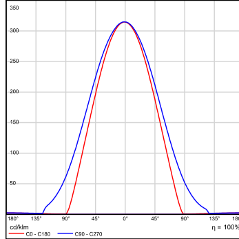
Işık Yayımlı 1 - Linear LVK Light emission 1 - Polar LVK
